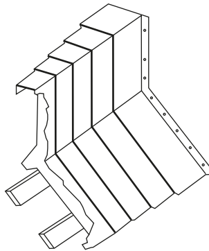
Schrägbettabdeckung Inclined bed cover
