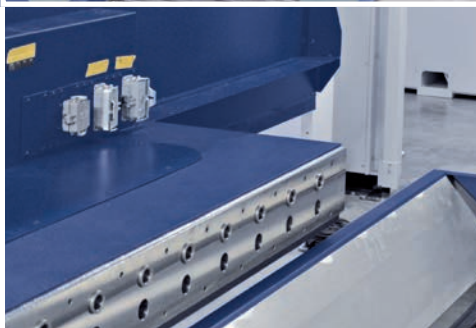
Fördersystem-Konfiguration an einer Laserschneidmaschine. Conveyor system configuration on a laser cutting machine.
