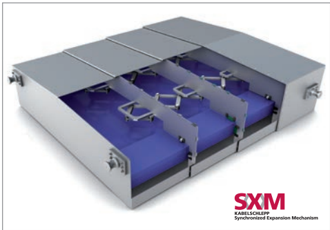
Teleskop-Abdeckung mit Scherenmechanik Telescopic cover with scissor mechanism
