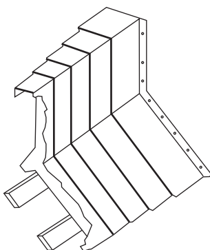
Schrägbettabdeckung Inclined bed cover
