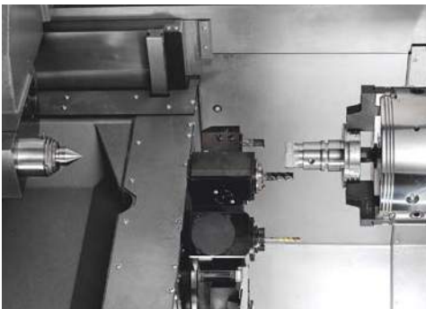
Arbeitsraumverkleidung an einer Universaldrehmaschine Work area cover for a universal lathe
