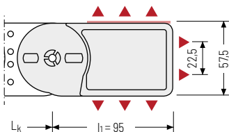
▲ Possibilités d'assemblage
