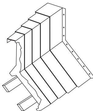
kryt šikmých loží inclined bed cover
