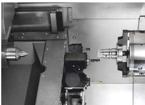
Obloženie pracovnej plochy na univerzálnom sústruhu Work area cover for a universal lathe
