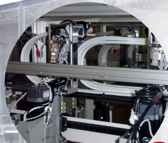
Freitragender CLEANVEYOR®
