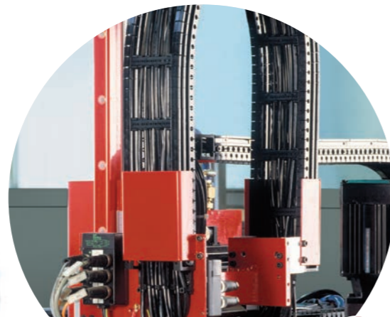
Vertikal angeordnete QUANTUM®-Energieführung
