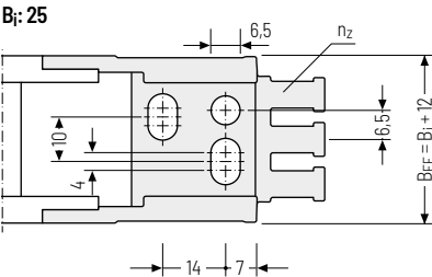
▲ Possibilités d'assemblage
